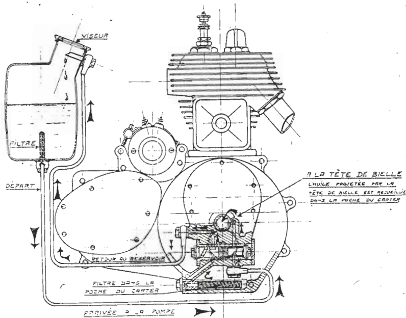
Schéma du graissage par circulation sur motocyclettés à carter sec.
