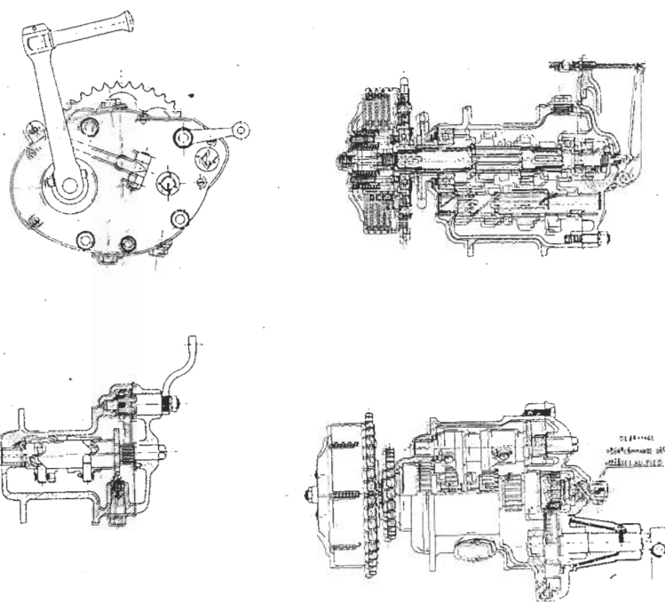
Boîte 4 vitesses « Terrot », type RAtt-VAtt.
