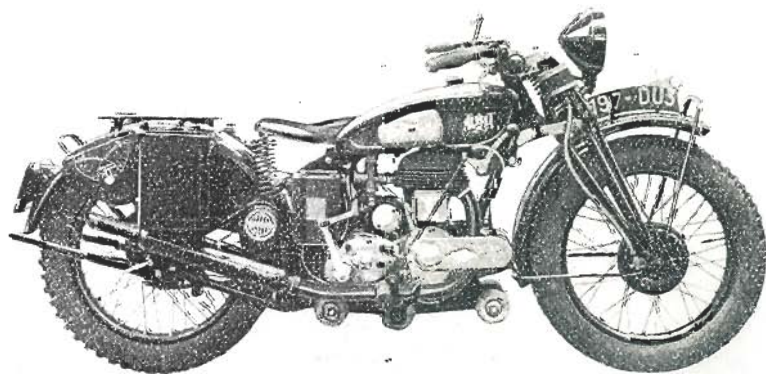
Vue de la moto type RAU, côté distribution.
