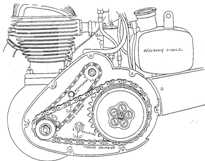
Schéma de graissage des chaînes sur moto RAT.
