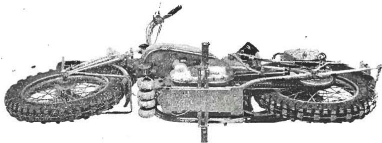
Vue en dessous de la moto type VAI montrant le train de rouleaux caoutchoutés.
