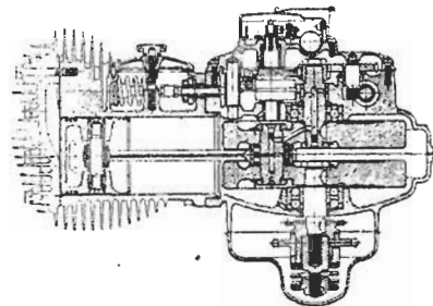
Moteur - TERROT 2, monocylindrique 500 cc.
