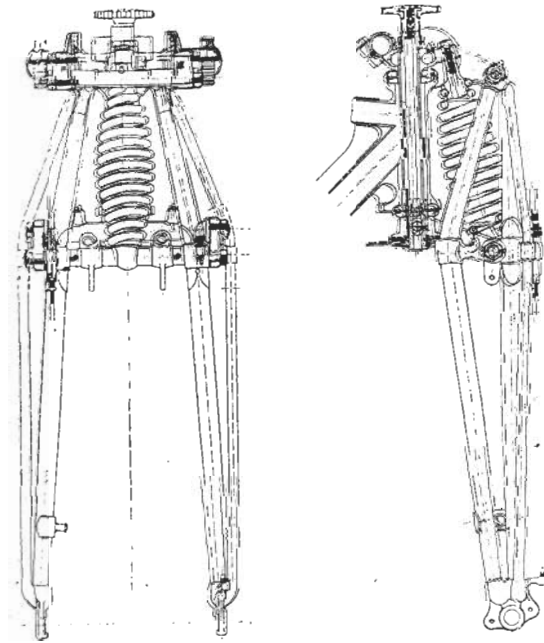
Fourche pour motos RAtt et VAtt Ressort central à la compression.
