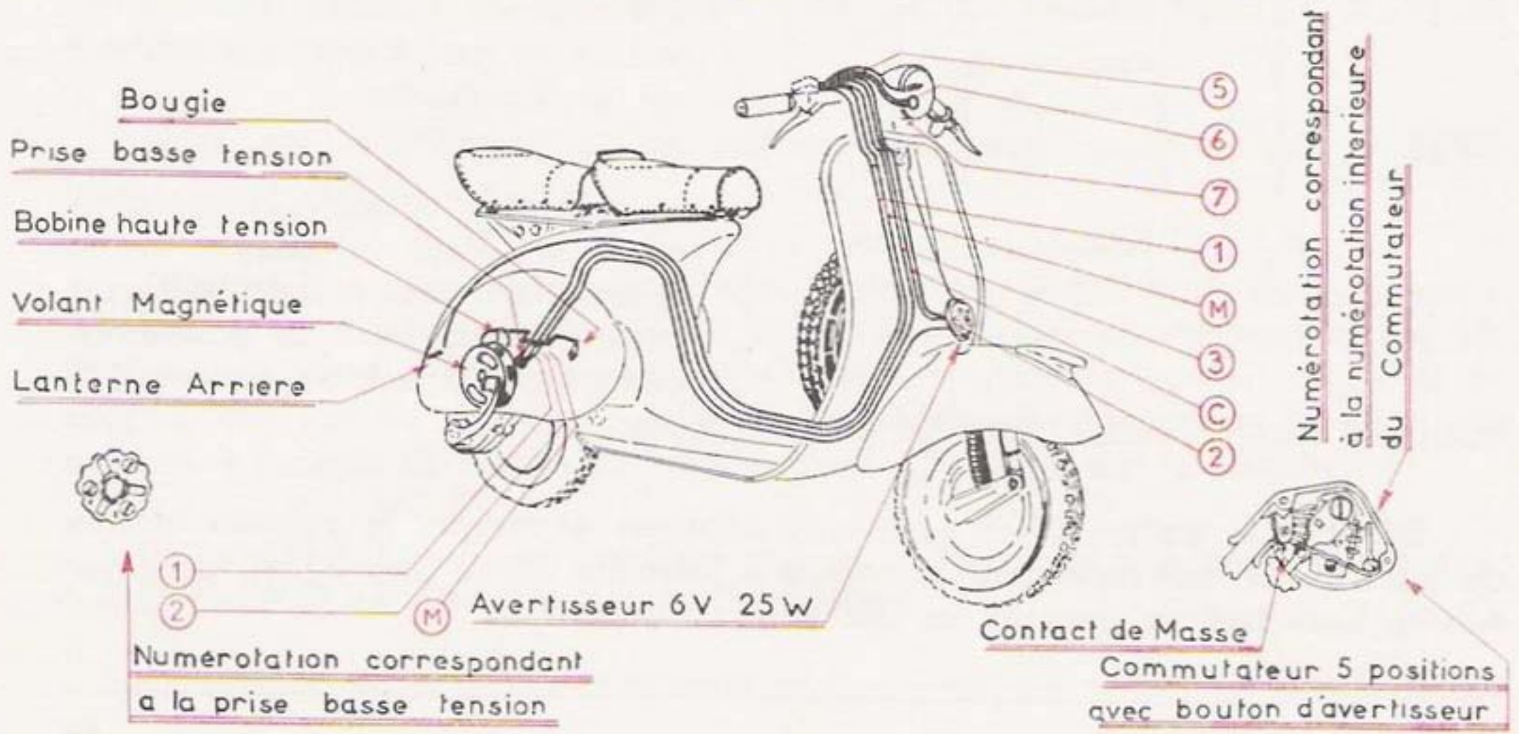
Fig. 7. — Schéma de l'implantation électrique.
