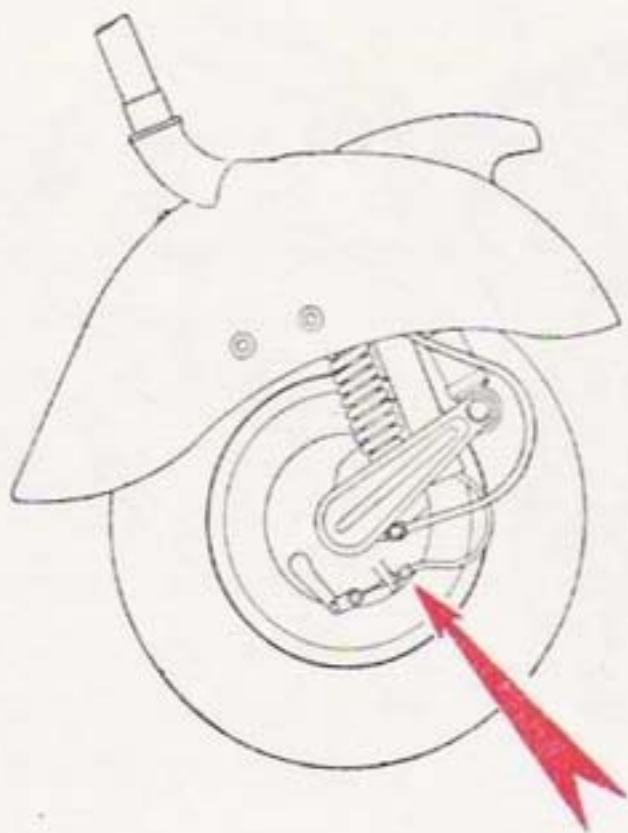
Fig. 12. — Réglage du frein avant.
