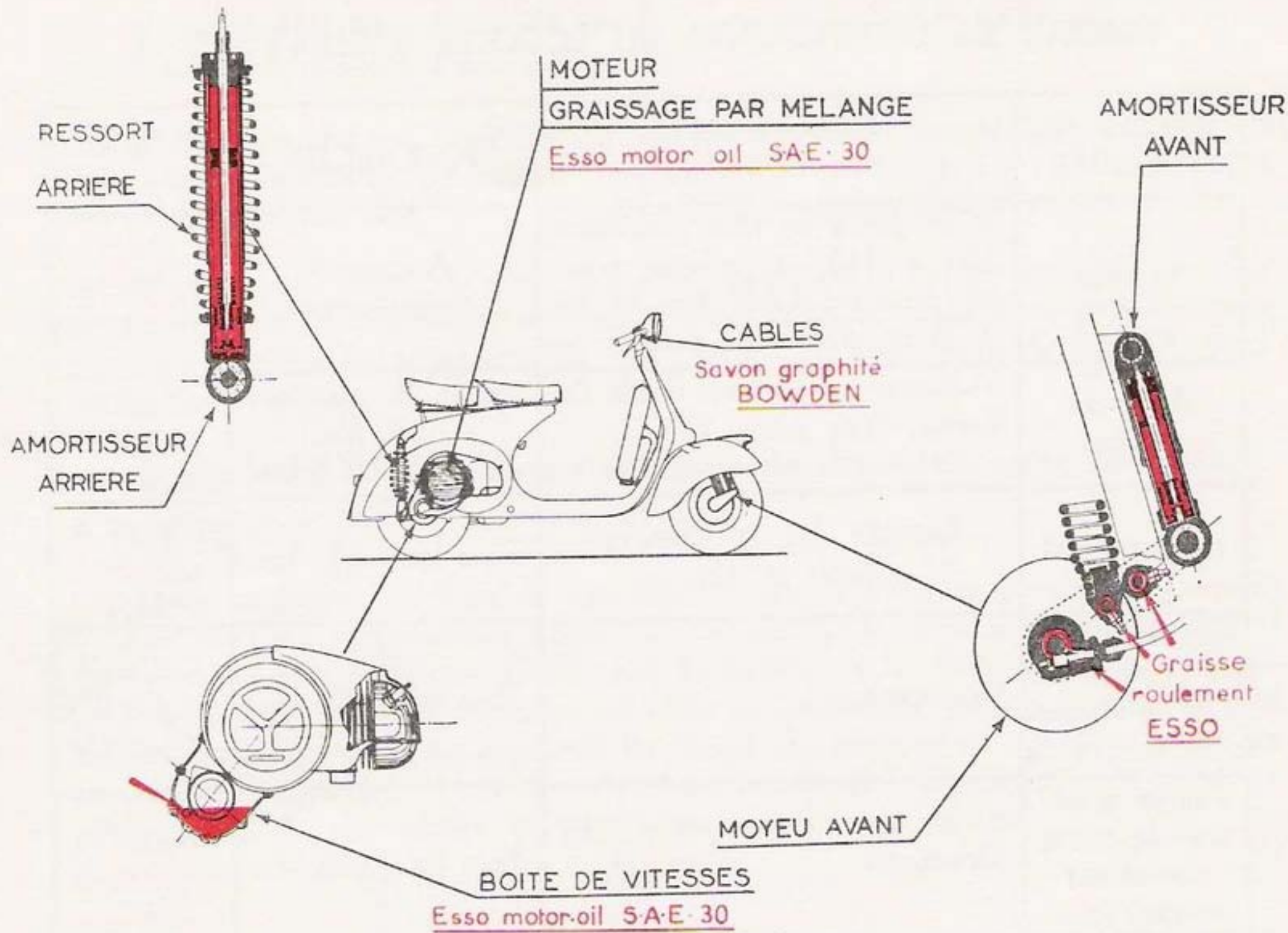
Fig. 17. — Graissage du Scooter.
