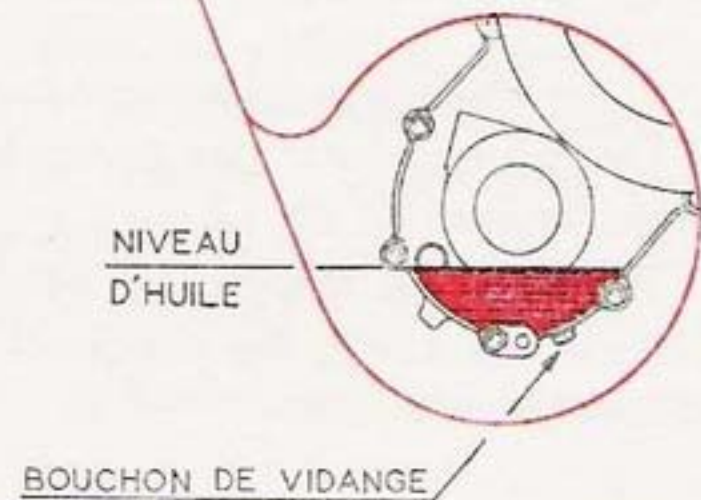
Fig. 14 Niveau de l'huile dans le carter.
