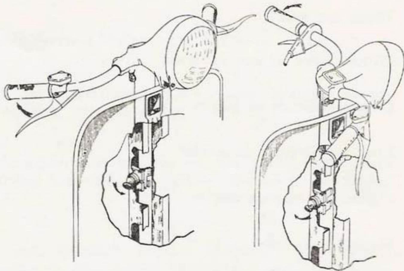
Fig. 3. — Dispositif antivol.
