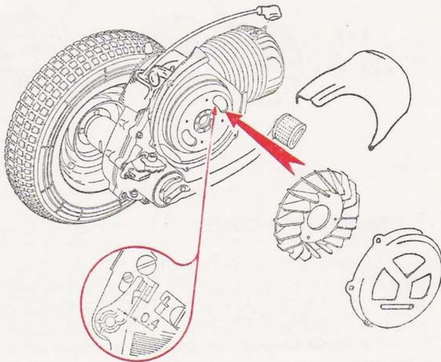
Fig. 15. — Contacts du rupteur.
